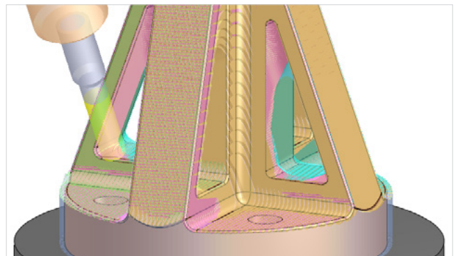
Comando di "Orientamento fresatura" automatico usando operazioni di sgrossatura a 3+2 assi. Il grezzo viene colorato in base all'orientamento. Le direzioni vengono definite automaticamente dal sistema
