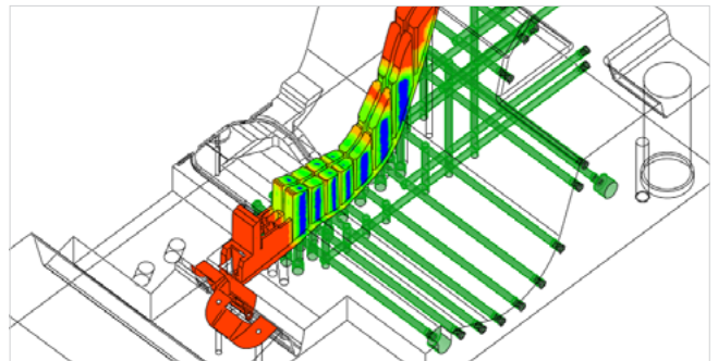
Mappa a colori delle distanze fra le facce delle parti e i canali di raffreddamento
